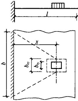
图 C. 0. 5-4 悬臂板上局部荷载的有效分布宽度
