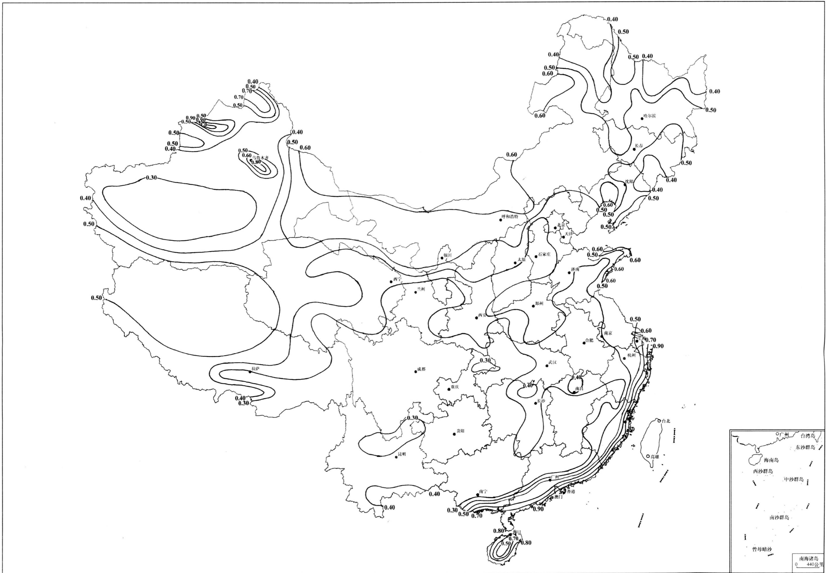
图 E. 6.3 全国基本风压分布图( \text{kN/m}^2 )
