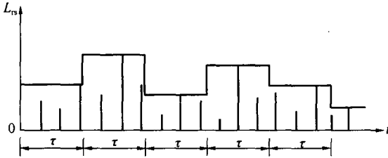
图 4 临时性活荷载随时间变化示意图
