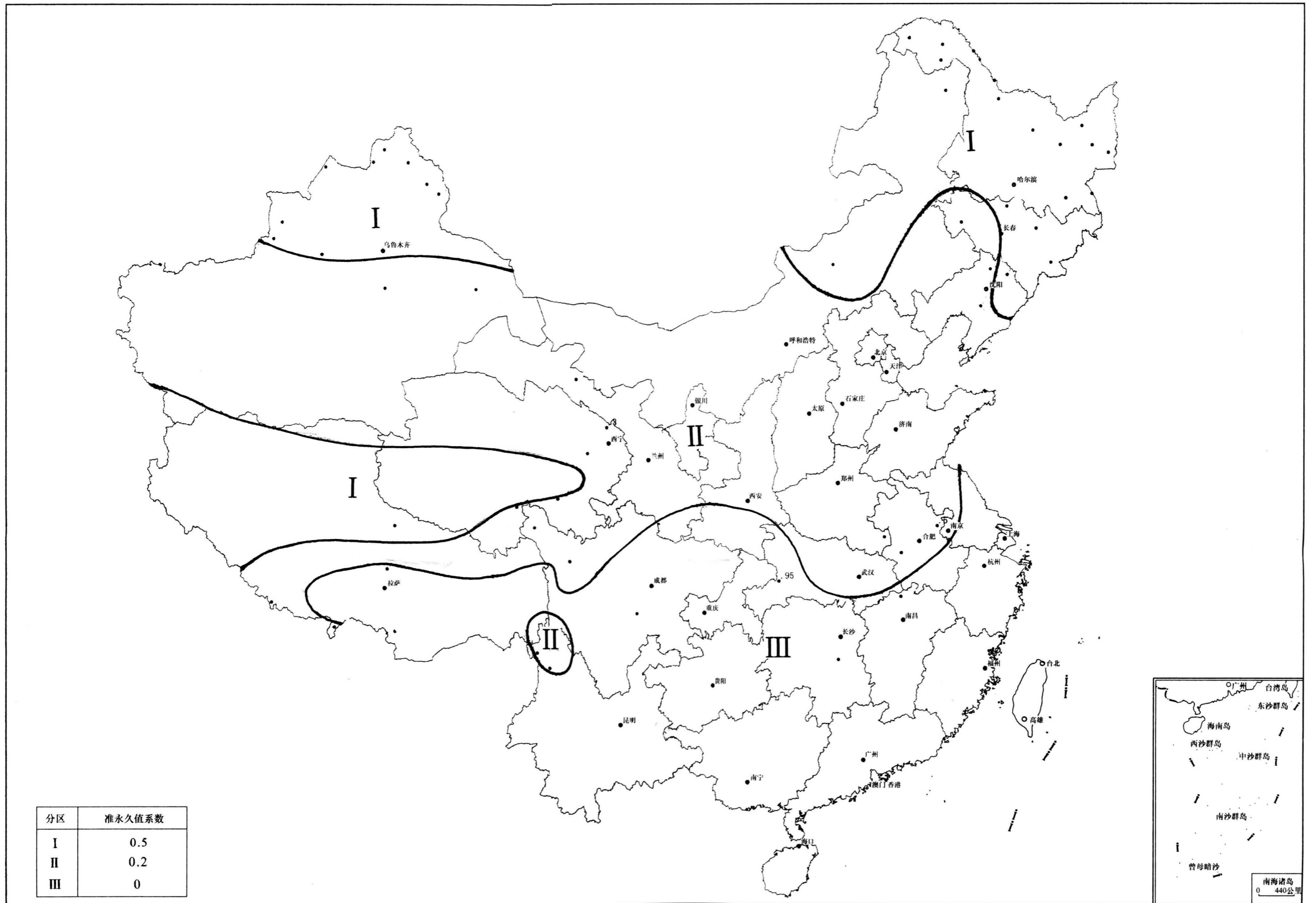
图 E.6.2 雪荷载准永久值系数分区图
