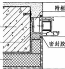
② 塑料门窗框、铝合金门窗框
