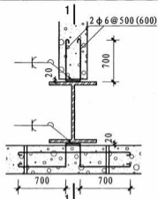
② 拉结筋 (非全长贯通)
