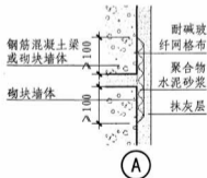
与圈梁构造柱接缝部位粘 贴玻纤网格布立面示例图
