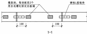
板材内墙弹性L型铁件连接构造详图
