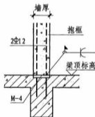
④ 框架梁(板)预埋件 (用于抱框)
