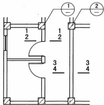
平面索引图
