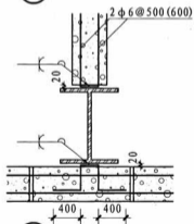
④ 拉结筋 (全长贯通)
