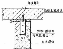
① 弹性L型铁件
