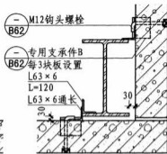
2 钩头螺栓法
