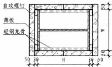
③ 工字形钢柱防火构造
