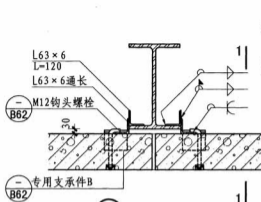
1 钩头螺栓法
