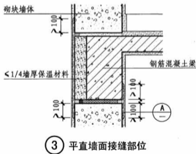
砌块墙体接缝部位防裂做法构造详图
