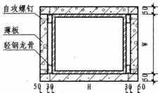
④ 方形钢柱防火构造
