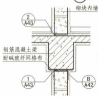
3-3 (无防水要求内墙)
