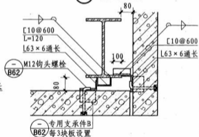
4 钩头螺栓法
